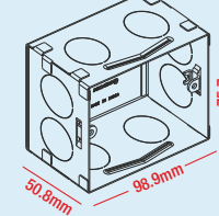
3 module 800173
