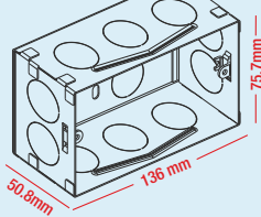
4 module 800174
