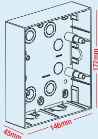
8 module (Vertical) 800187
