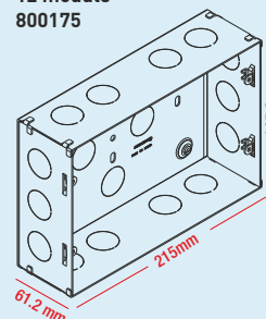
12 module 800175
