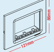
3 module 800163
