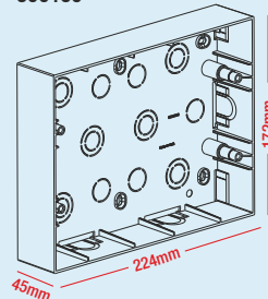
12 module 800185
