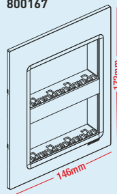
8 module (Vertical) 800167
