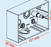
3 module 800183
