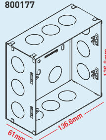
8 module (Vertical) 800177
