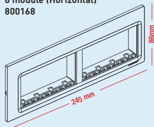
8 module (Horizontal) 800168
