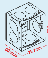
1 & 2 module 800172
